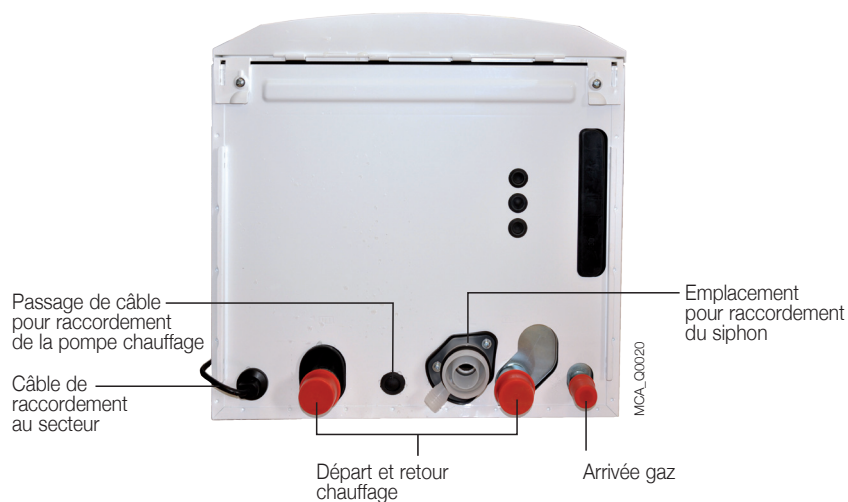
Vue du dessous de la chaudière
