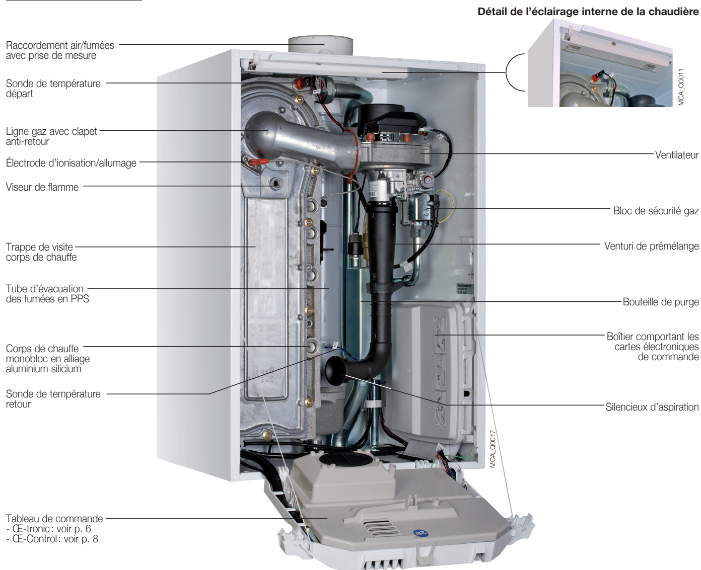
Détails corps de chauffe en alliage aluminium/silicium
