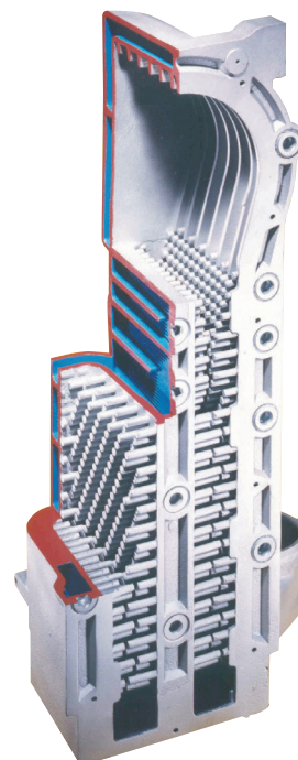
Détails corps de chauffe en alliage aluminium/silicium
